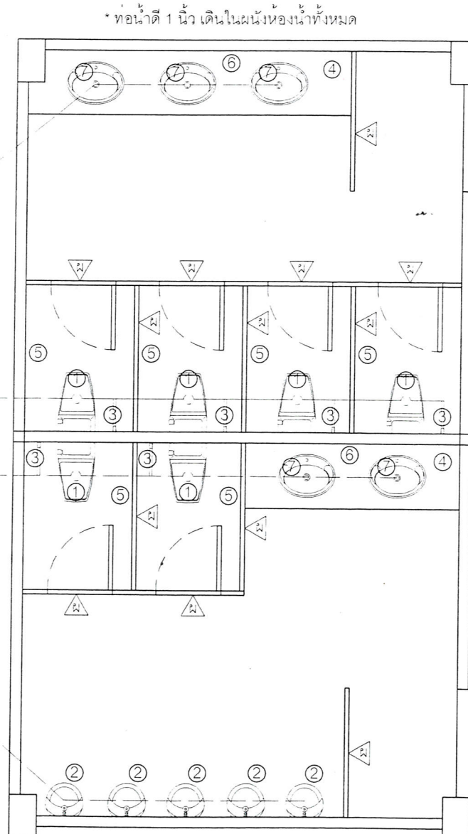
แปลนระบบประปา
